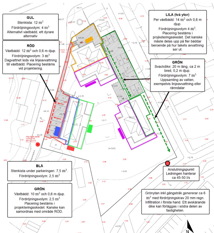
Bild 10. Schematisk bild över dagvattenhanteringen. Underlags bild Forsgren Etzler Arkitekter 2023.
