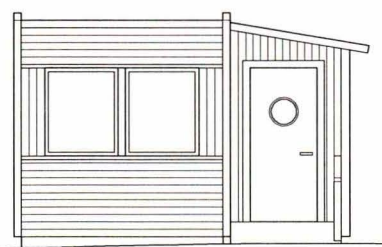
FASAD MOT NORR
