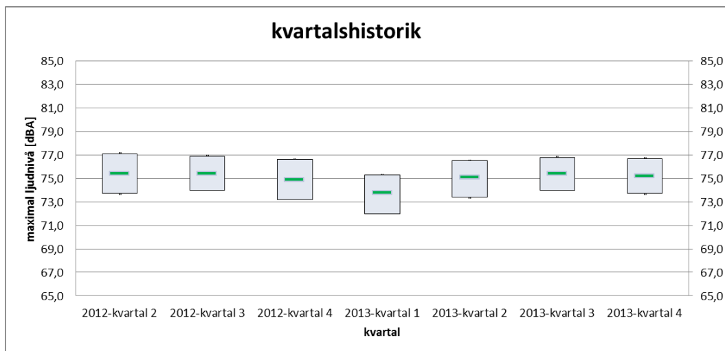
Figur 7 Jämförelse av registrerade maximala nivåer för landningsrörelser på bana 01L under varje kvartal i boxdiagram. Lådan innesluter 50% av all mätdata under respektive kvartal och grönt streck visar medianvärde av samtliga registrerade mätvärden.
