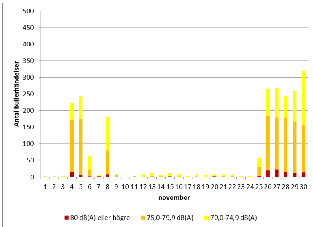
Figur 3 Antal bullerhändelser i intervaller om 5 dB i november 2012.
