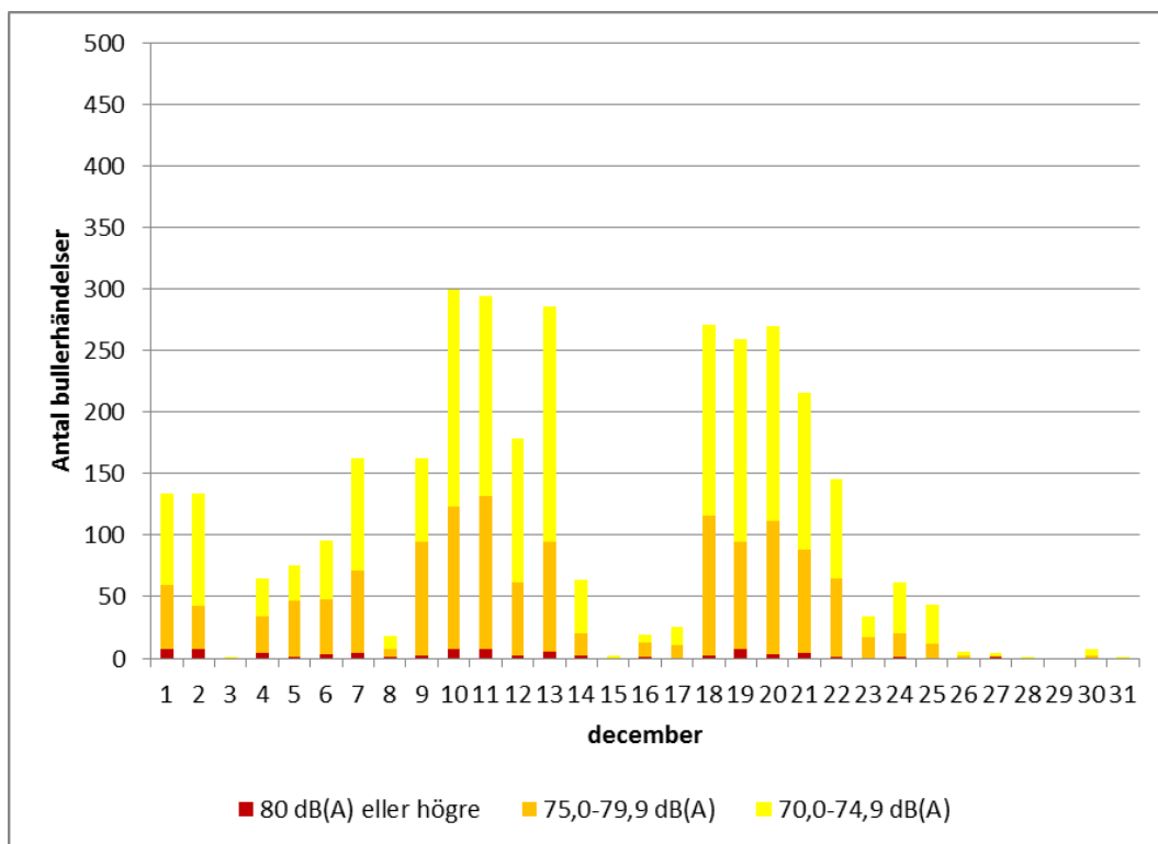
Figur 4 Antal bullerhändelser i intervaller om 5 dB i december 2012.
