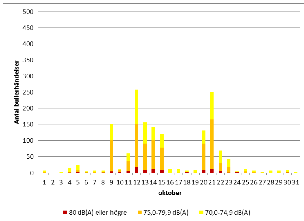
Figur 2 Antal bullerhändelser i intervaller om 5 dB i oktober 2012.
