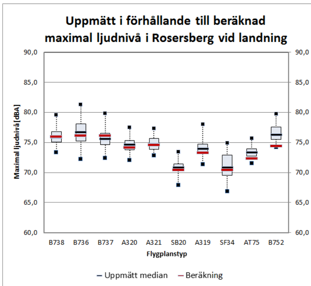
Figur 4 Låddiagram för de tio vanligaste flygplanstyperna som landar på bana 01L under tredje kvartalet 2015.
