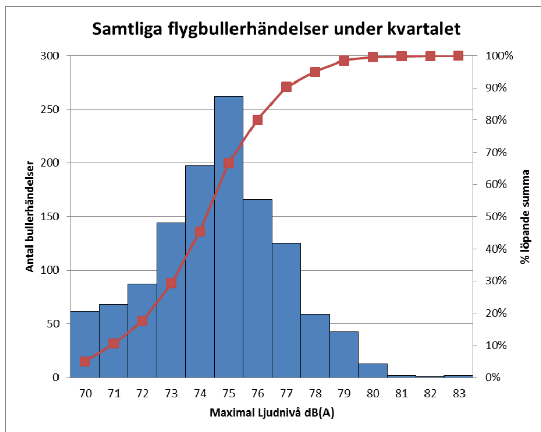
Figur 2 Histogram redovisande antal flygbullerhändelser per ljudnivåintervall från 70 dB(A) och högre i steg om 1 dB. Stapeln för 70 dB(A) omfattar maximala ljudnivåer från 70 – 70,9 dB(A) osv. Löpande summa i procent redovisas som röd linje med förklaring längs den sekundära y-axeln.
