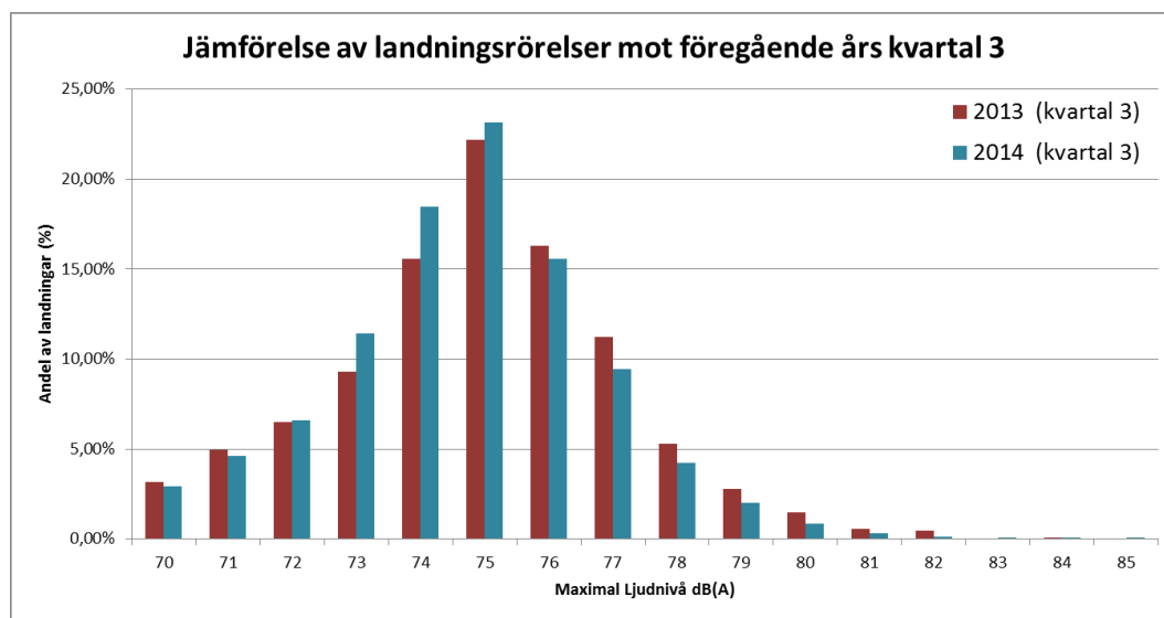
Figur 6 Jämförelse av landningspassager för årets kvartal 3 (2014) mot föregående års kvartal 3 (2013). Andelen mätningar mellan 70 till 85 dB(A) visas i procentheter.
