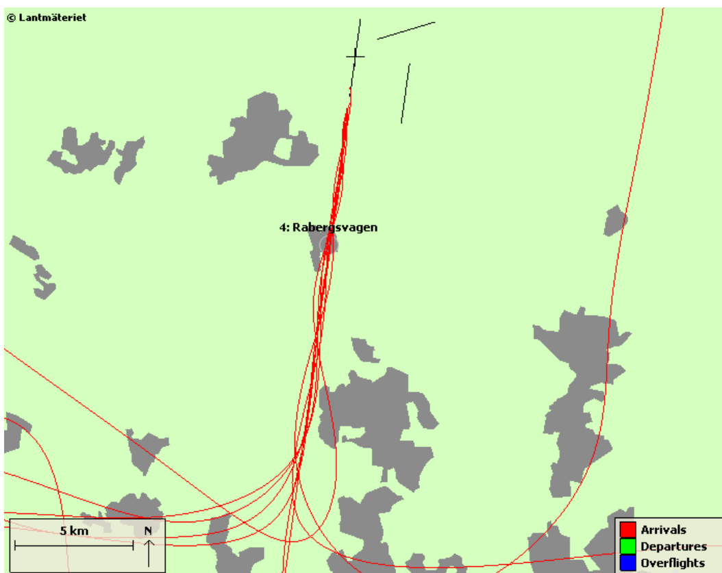
Figur 10 Radarspår illustrerande de tio högst registrerade maximala ljudnivåer under tredje kvartalet 2014.
