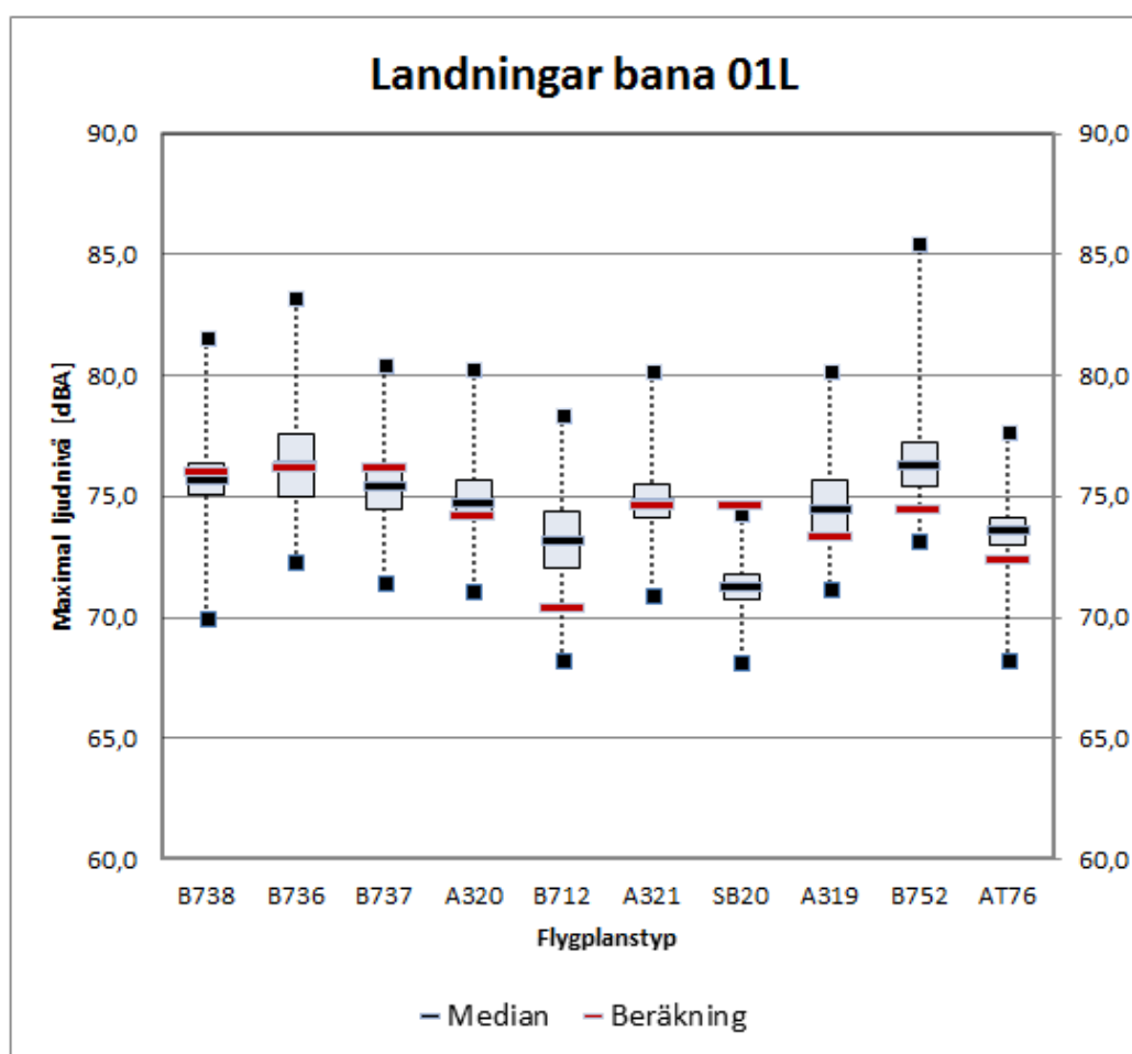
Figur 9 Låddiagram för de tio vanligaste flygplanstyperna som landar på bana 01L under tredje kvartalet 2014.
