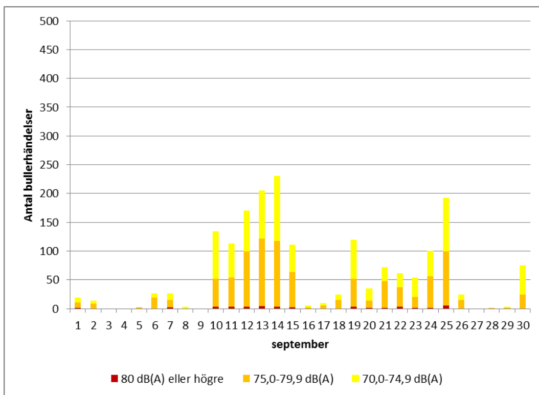
Figur 4 Antal bullerhändelser i intervaller om 5 dB i september 2014.
