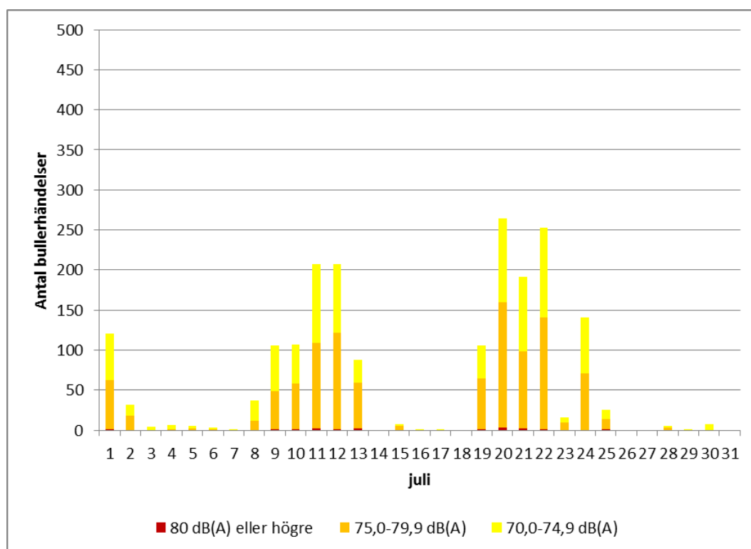
Figur 2 Antal bullerhändelser i intervaller om 5 dB i juli 2014.
