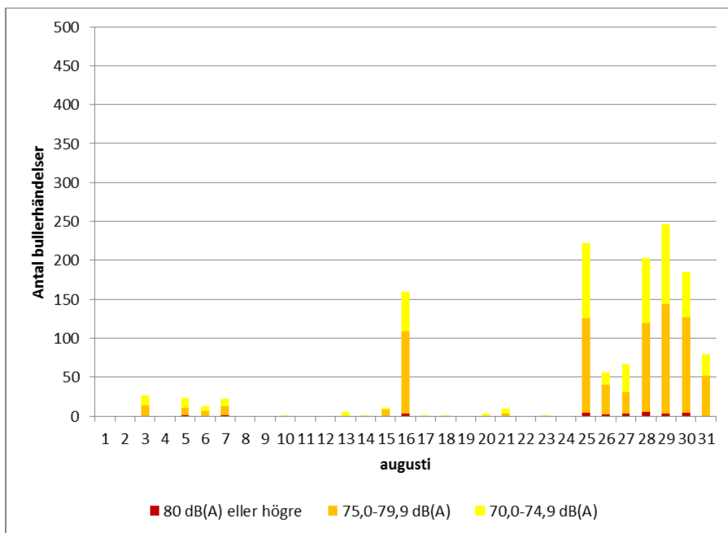
Figur 3 Antal bullerhändelser i intervaller om 5 dB i augusti 2014.
