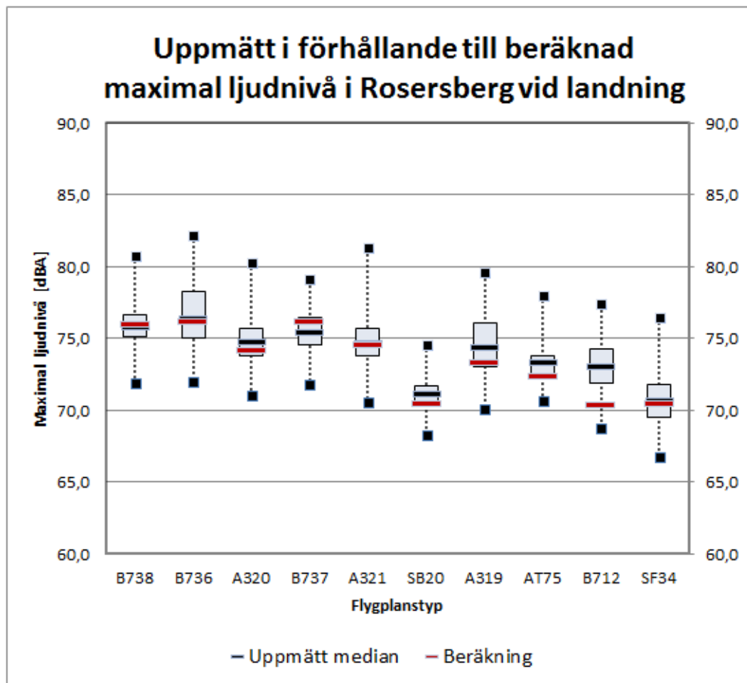
Figur 7 Låddiagram för de tio vanligaste flygplanstyperna som landar på bana 01L under andra kvartalet 2015.
