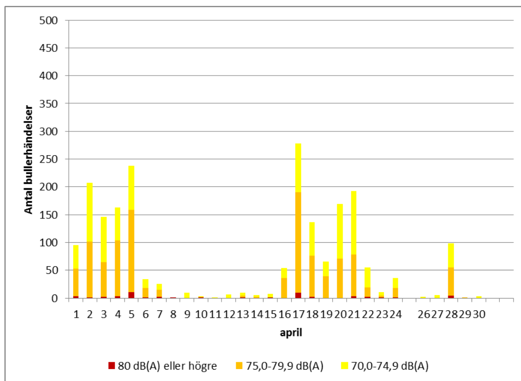
Figur 2 Antal bullerhändelser i intervaller om 5 dB i april 2015.
