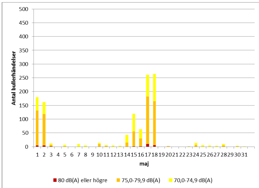
Figur 3 Antal bullerhändelser i intervaller om 5 dB i maj 2015.
